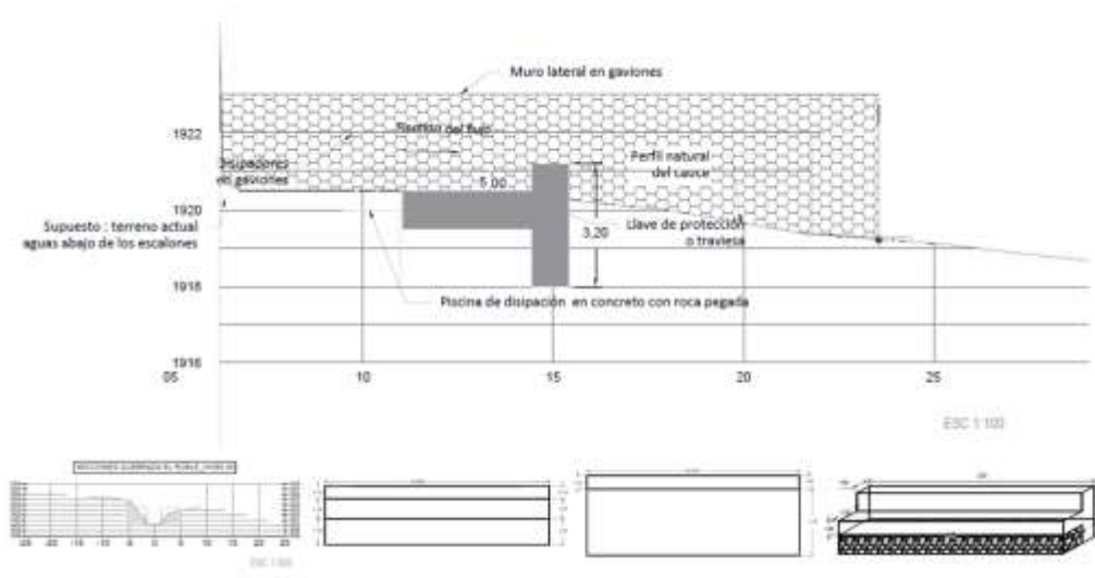
Ilustración 1. detalle de las traviesas a construir
