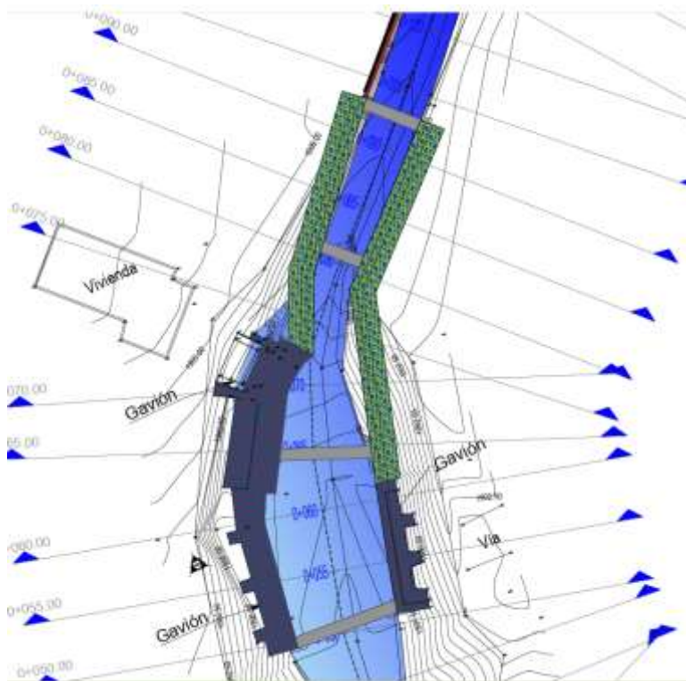
Ilustración 3. intervención a realizar en la Quebrada La Ceja, fase.
