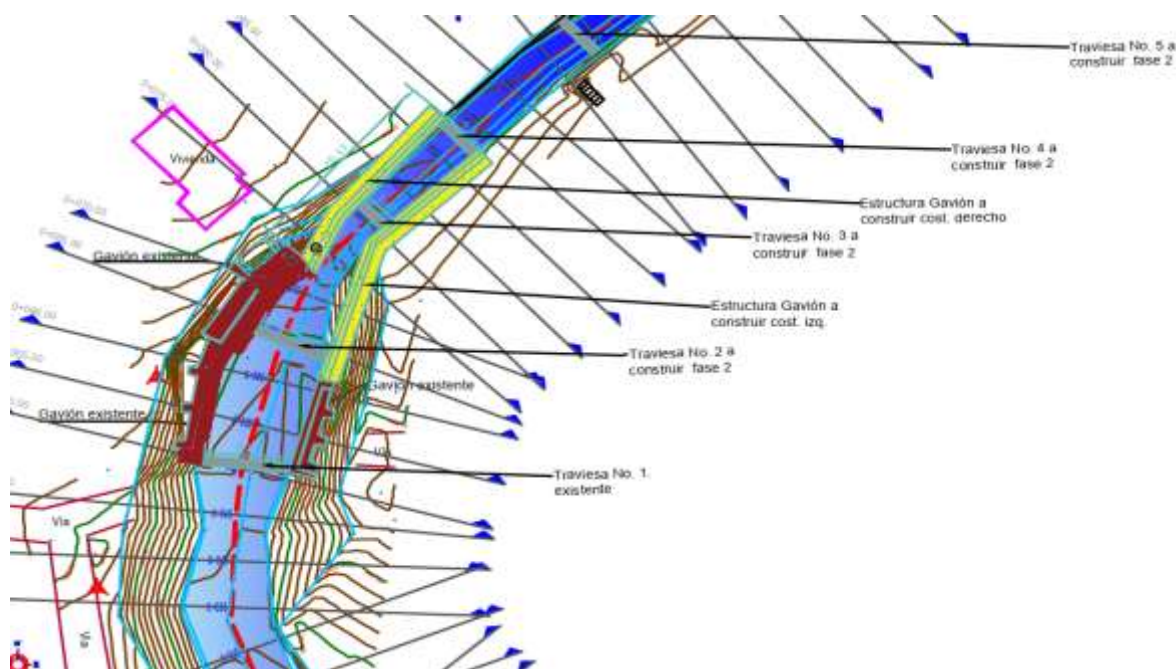
Ilustración 2. Obras propuestas para la segunda fase de la intervención
